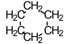
Cyclohexan
