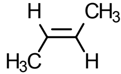
(2 E )-2-Buten
