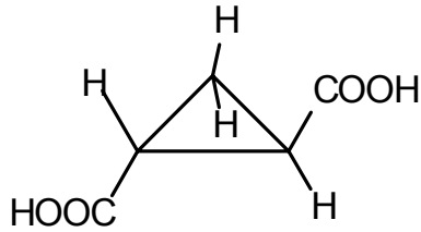
cis-Cyclopropanedicarbonsäure Smp: 139°C
