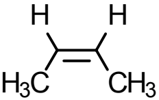
(2 Z )-2-Buten
