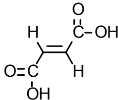
Fumarsäure Smp: 287°
