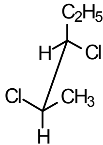
Sägebock -
